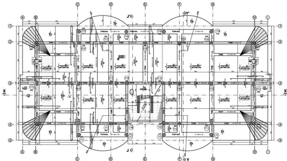
Pianta carpenteria edificio Via Morbegno (Roma)
